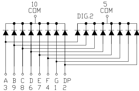
H. WCN2-XX30XX-A11
