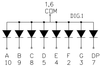
G. WCN2-XX30XX-A11
