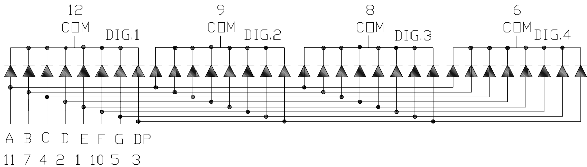
H. WCN4-0030XX-C11
